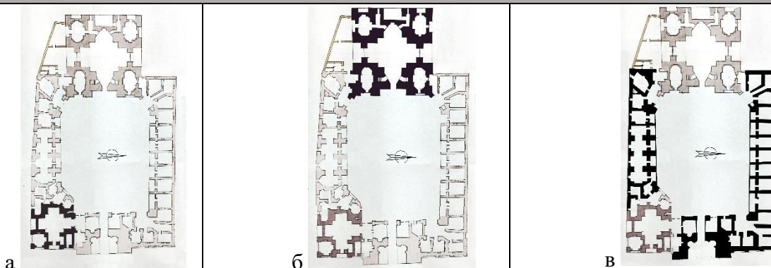
а) Строительство центрального мавзолея «Безымянный»; б) Строительство мавзолея «Суюнидж-хан»; в) Строительство портала и худжр. Вариант восстановления.
