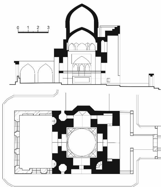
План мавзолея Каффаль Шаши. Источник: Булатова, Маньковская, 1983.
