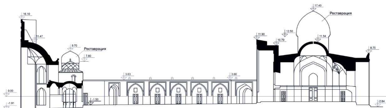
Проект реконструкции медресе Барак-хана, выполненный в 1956 г. Разрез медресе. Источник: Архив Глав НПУ.
